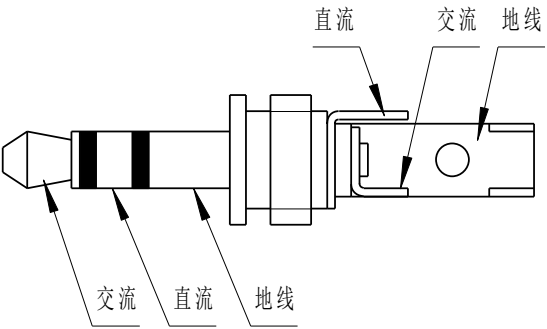
图 24 模拟输出插头的连接
