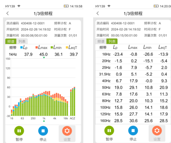
图 20 1/3 倍频程测量
