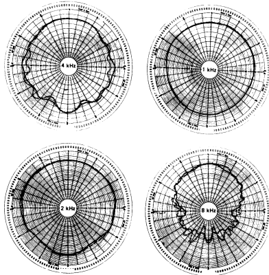
图 2 在不同频率下的指向特性
