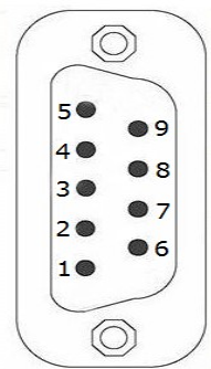
b) DB9 型母头背面引脚
