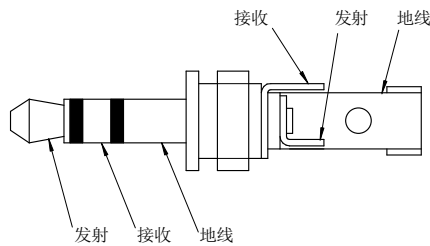
a) 双声道插头
