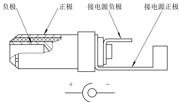
图 9 外接电源插头的极性 & 接线
