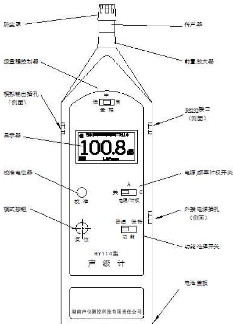
图 6 HY114 外形图
