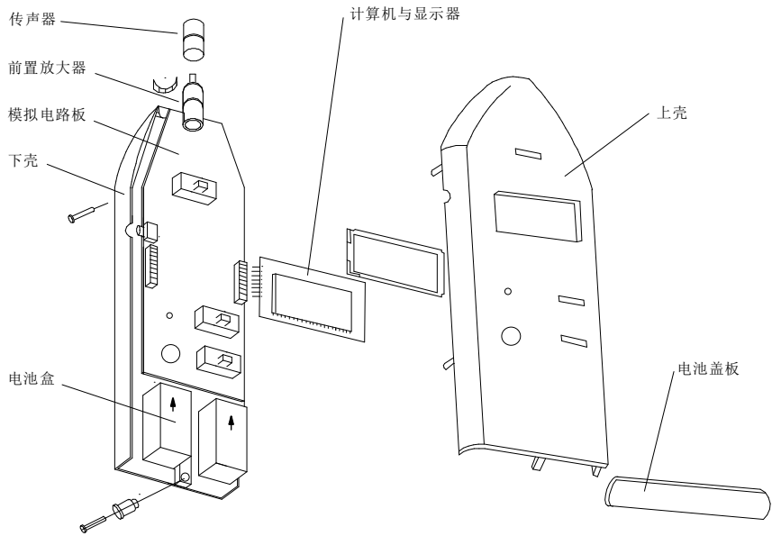
图 5 结构简图
