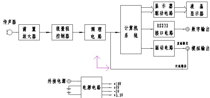
图 4 原理性方框图
