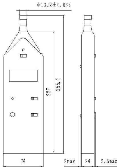
图 3 外形尺寸图
