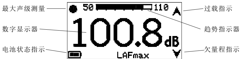
图 7 显示器的字符
