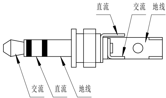
图 10 模拟输出插头的接线
