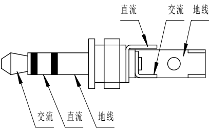
图 10 模拟输出插头的连接
