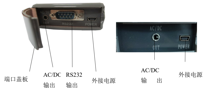
图4 输出接口图
