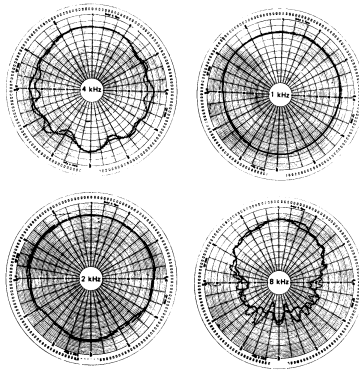
图 2 声级计在不同频率下的指向特性
