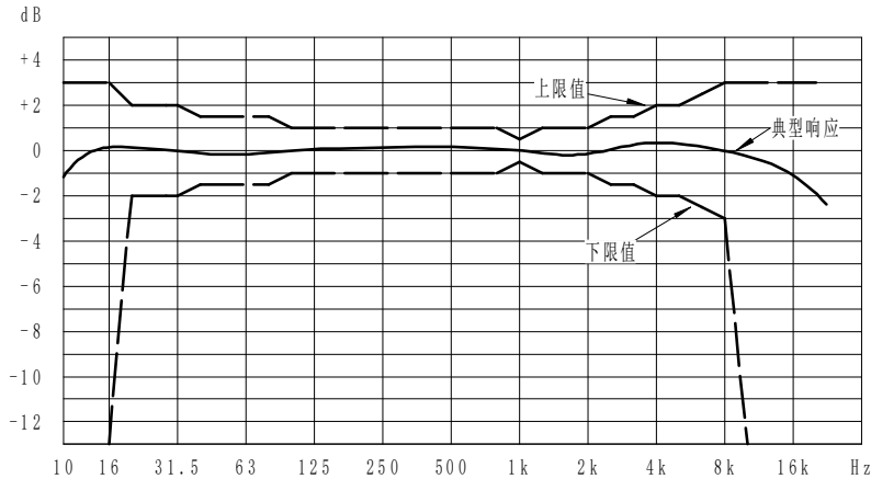
图 1 测量传声器的典型频率响应
