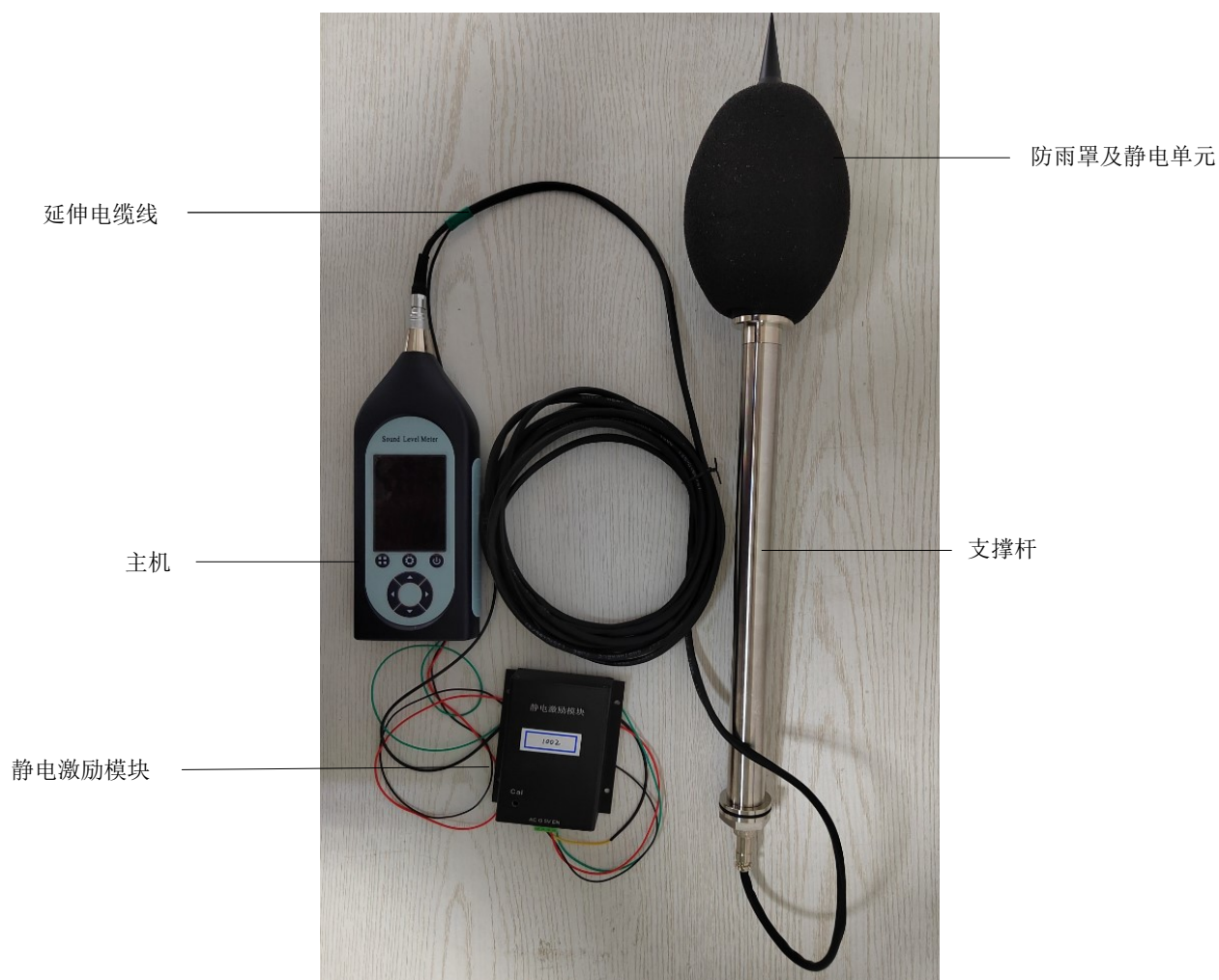
图 2 HY128B 型多功能声级计（户外）的外形图
