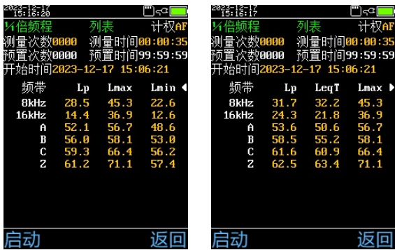
图 15 1/1 倍频程界面
