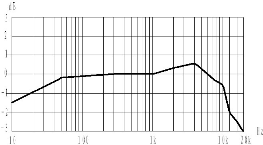
图 1 HY205 型传声器的典型频率响应
