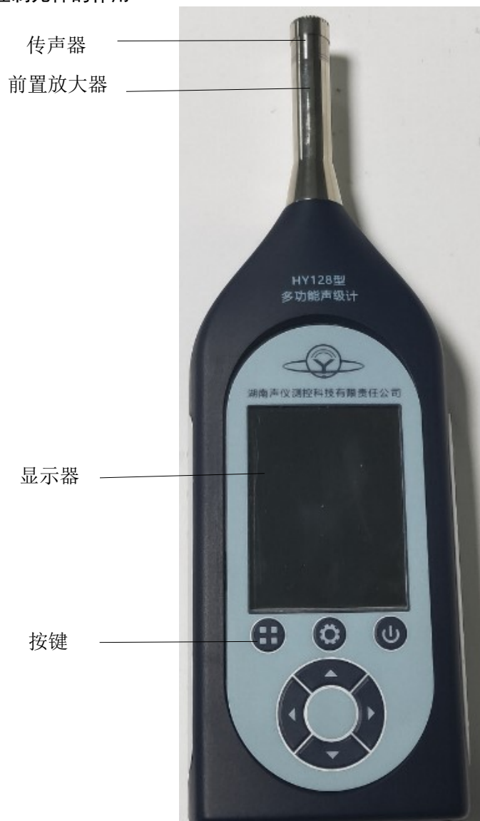
图 2 外形图
