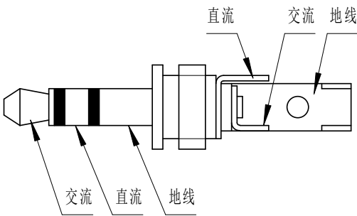
图 11 模拟输出插头的连接
