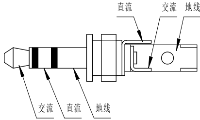
图 10 模拟输出插头的连接
