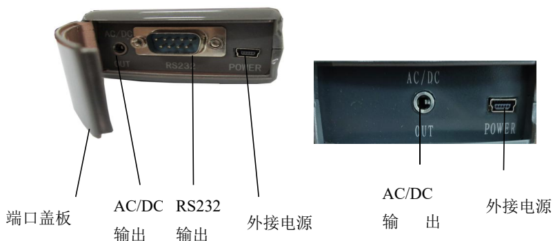
图 4 输出接口图
