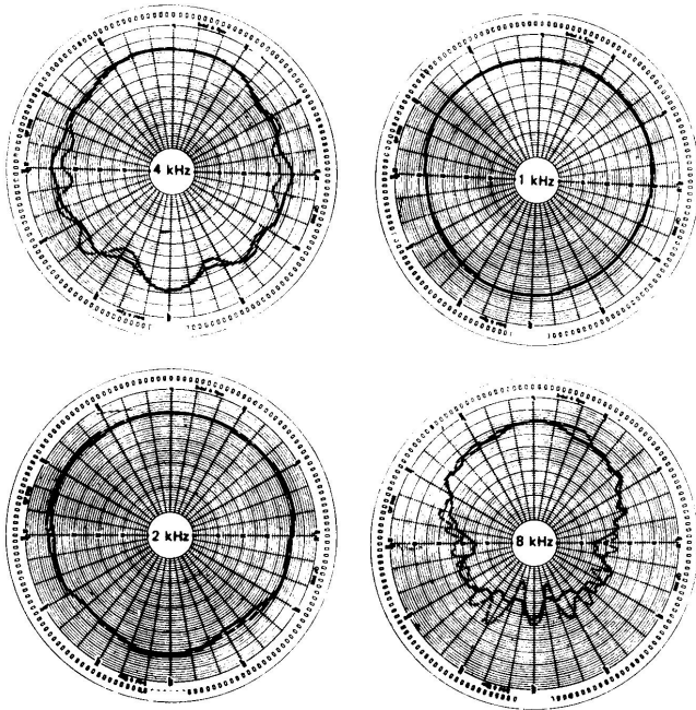
图 2 声级计在不同频率下的指向特性
